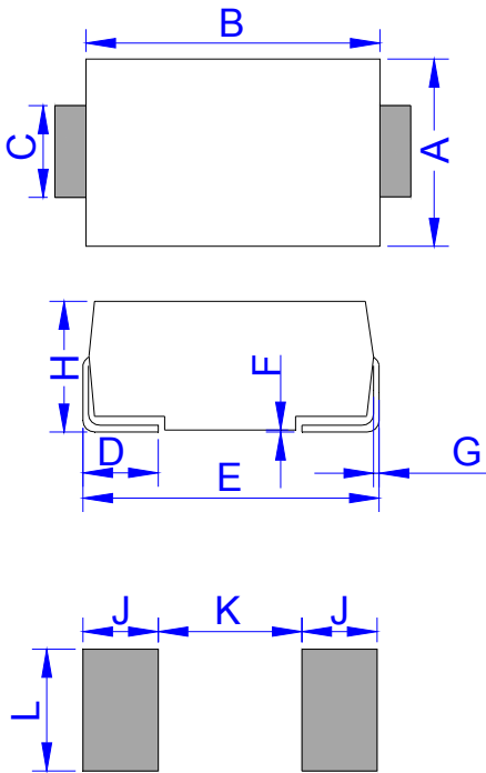
DO-214AB (SMC)
